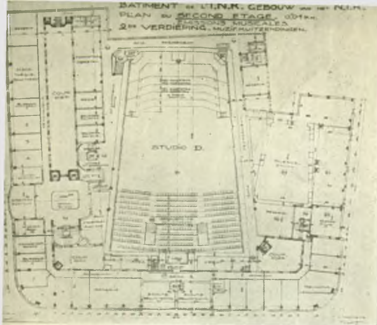
PLAN DER 2 e VERDIEPING VAN HET GEBOUW VAN HET N.I.R. HET GROOT AUDITORIUM (15.000 M3).
